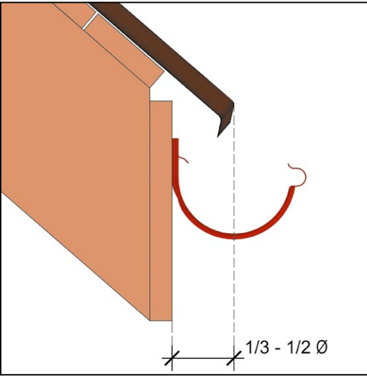
Рис. 4 Схема установки желоба водосточной системы Döcke
