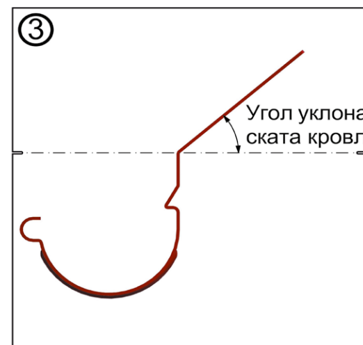
Рис. 8 Загиб карнизного крюка при помощи кронштейногиба
