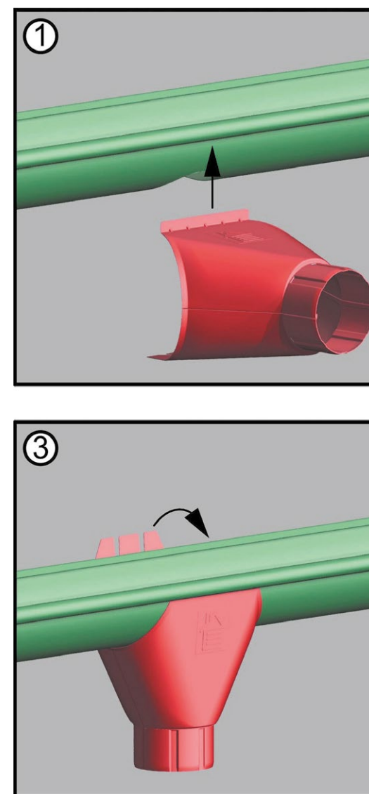
Рис. 17 Установка воронки
