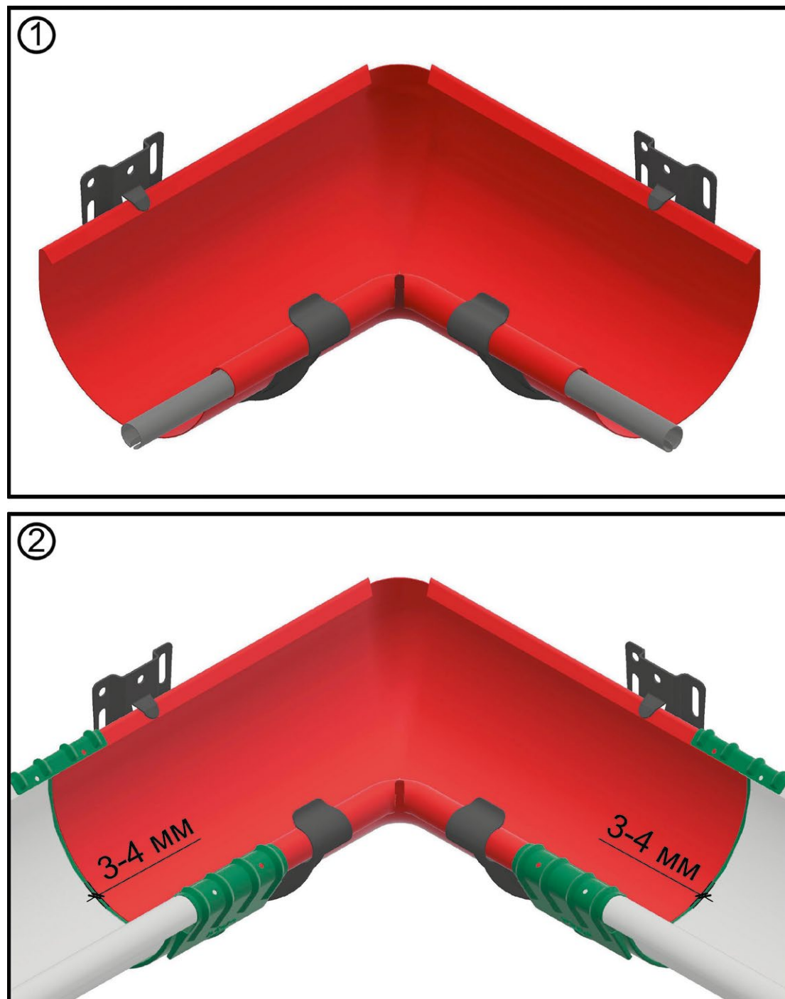
Рис. 16 Установка угловых элементов
