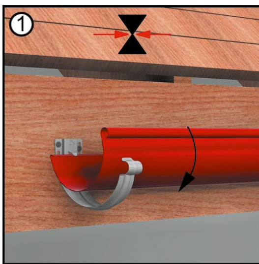
Рис. 14 Установка желоба на кронштейны.
