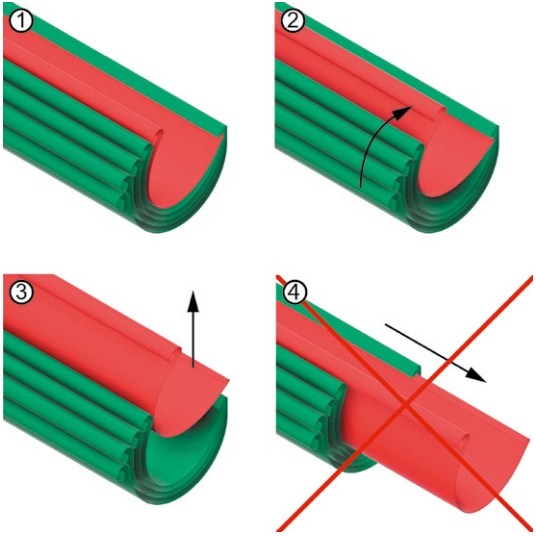
Рис. 1 (1-3) Схема распаковки металлических желобов водосточной системы Döcke. Рис. 2 (4) Неверная распаковка металлических желобов водосточной системы Döcke
