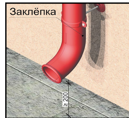
Рис. 21 Установка отвода трубы
