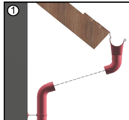
Рис. 20 Организация перехода от карнизной части здания к его фасаду
