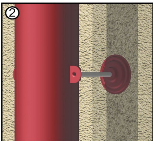
Рис. 19 Монтаж хомутов
